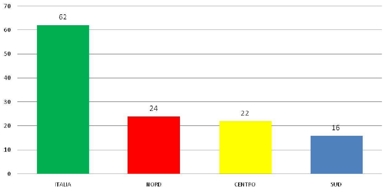
Impianti produzione CDR per macroarea attivi nel 2008 (fonte: Ispra)
