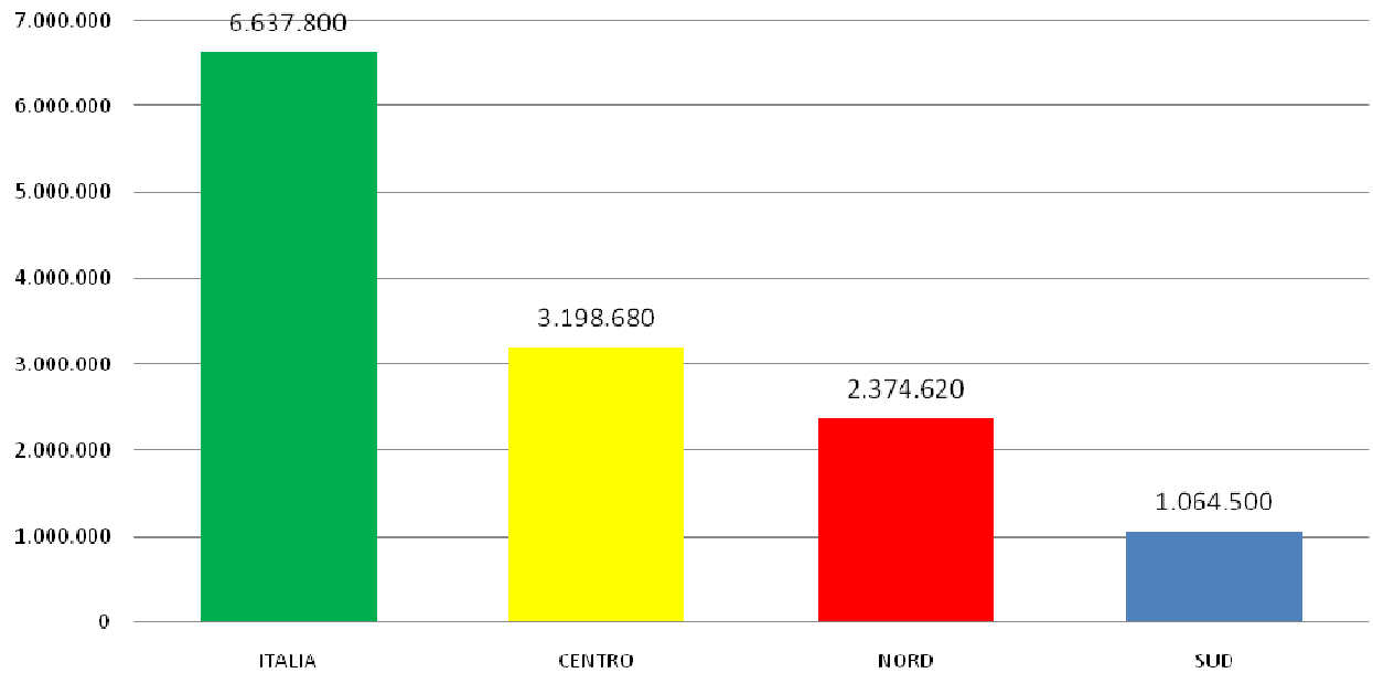
Potenzialità impianti produzione CDR per macroarea nel 2008 (t/a) (fonte: Ispra)
